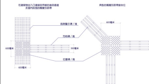
圖 7-4 觸覺顯示帶的規格
