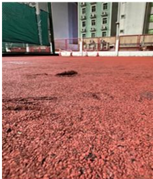
圖二：地面的地膠出現溶化
